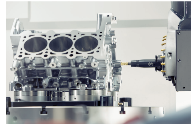
Zylinderkopfbearbeitung mit dem TENDO Slim 4ax
